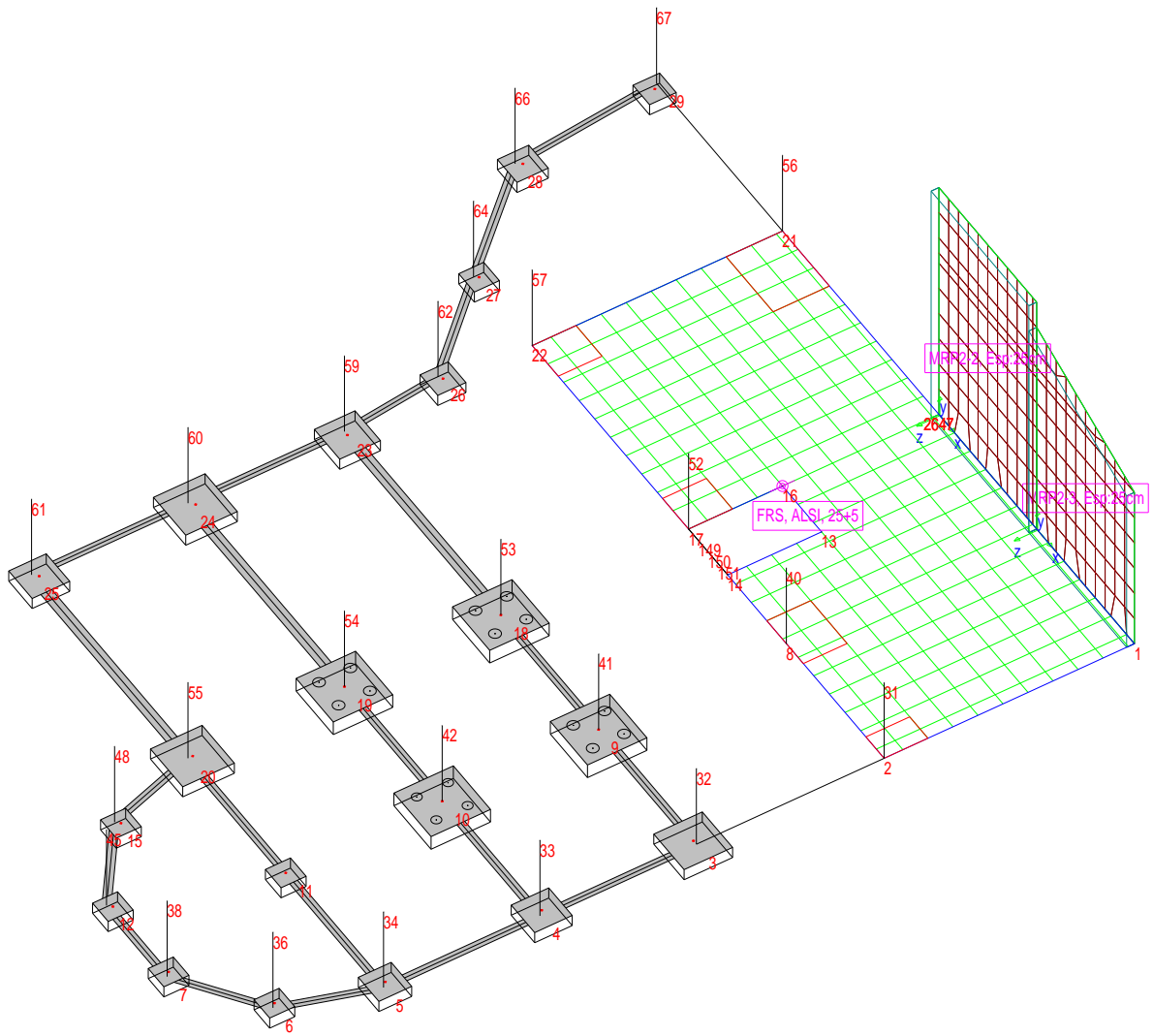
Reacciones. Ejes generales, Hormigón, E.L.U., sin mayorar
